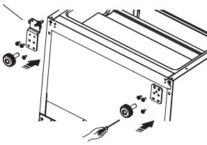
Onderstescharnieronderdeel (links)
